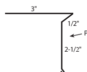
22b 6" T-STYLE DRIP EDGE FT02
